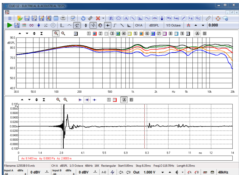
MLS & LogChirp
